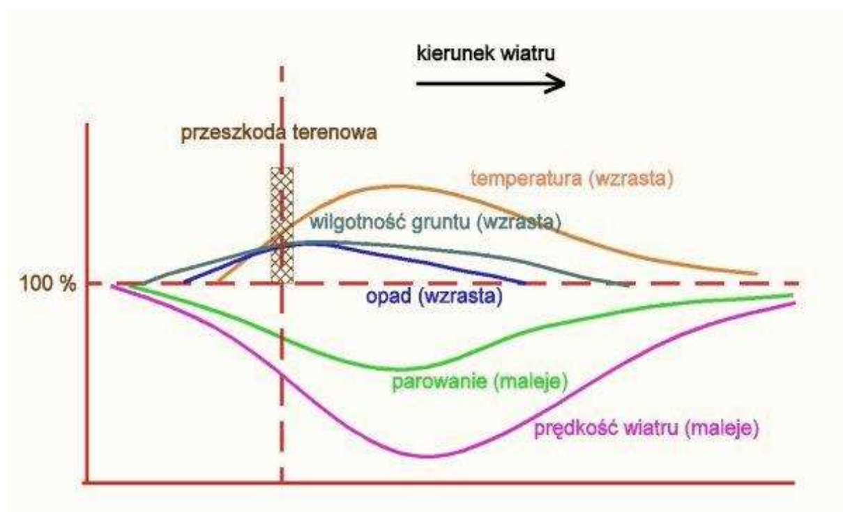
Rys. 9. Zmiany parametrów fizycznych wywołanych przez przeszkodę terenową
