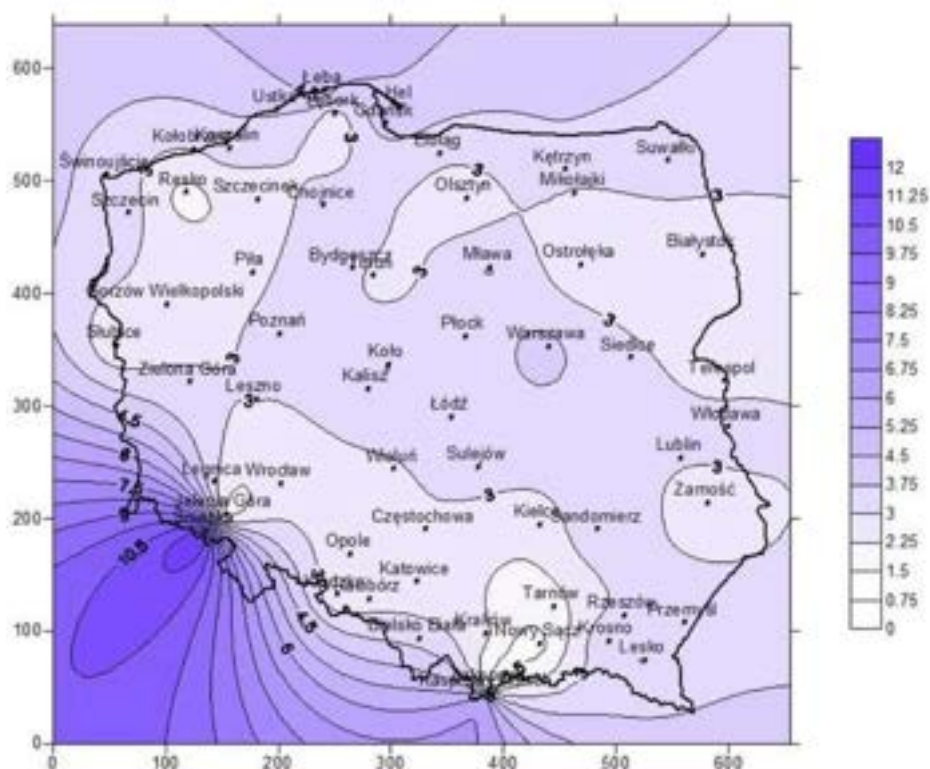
Rys. 3. Mapa średniorocznych wietrzności Polski [m/s]
