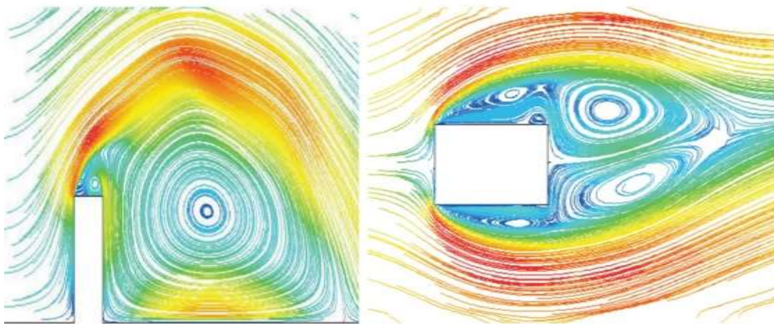
Rys. 8. Schemat działania prądu powietrza wokół przeszkody umieszczonej w poziomym przepływie, widok z boku i z góry
